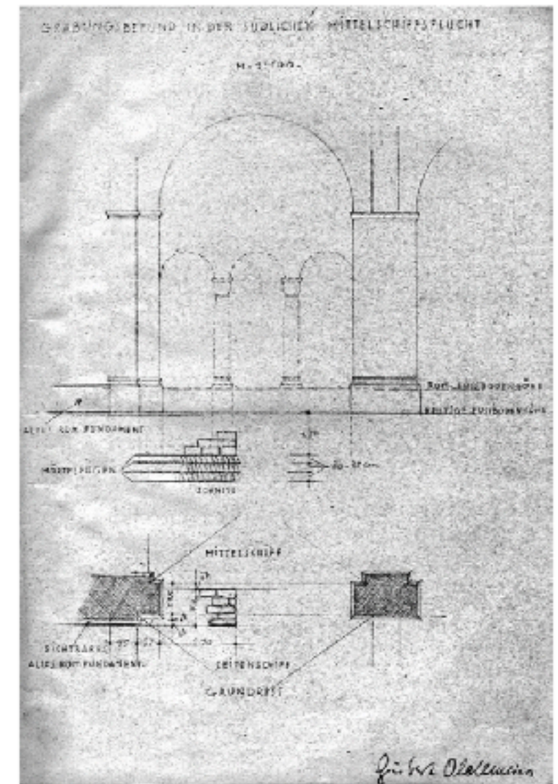
Grabungsbefund in der südlichen Mittelschiffsflucht, M 1:200. – OLDEMEIER 1942,
